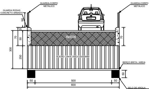
SEÇÃO LONGITUDINAL (CORTE A-A) ESCALA 1/75
