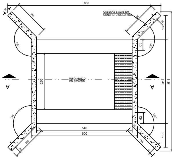
PLANTA BAIXA - TUBO ARMCO ESCALA 1/75
