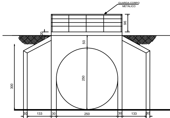
VISTA FRONTAL ESCALA 1/75
